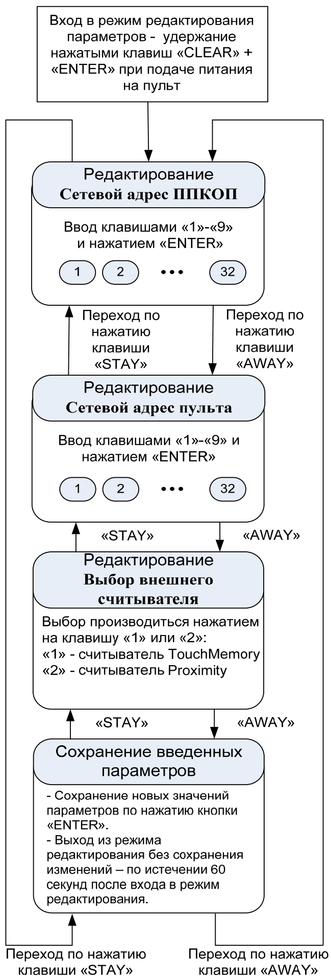
Рисунок 8 – Цикл редактирования параметров пульта.
