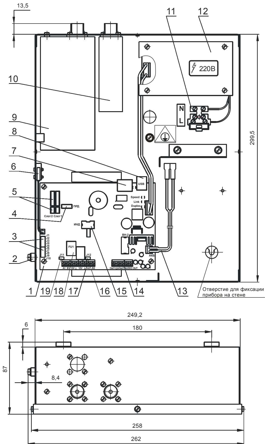
Рисунок 2 - Размещение узлов в кожухе ретранслятора
