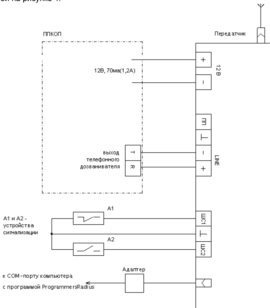
Рисунок 4 – Схема подключения передатчика МС
