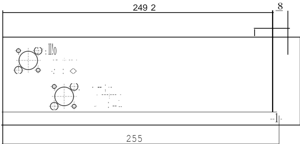
ПЛИСУНОК А.1 - рабапiiiTHble III yCTaHOBO4Hble pa3Mepbl np1116opa «npOTOH-8/16»
