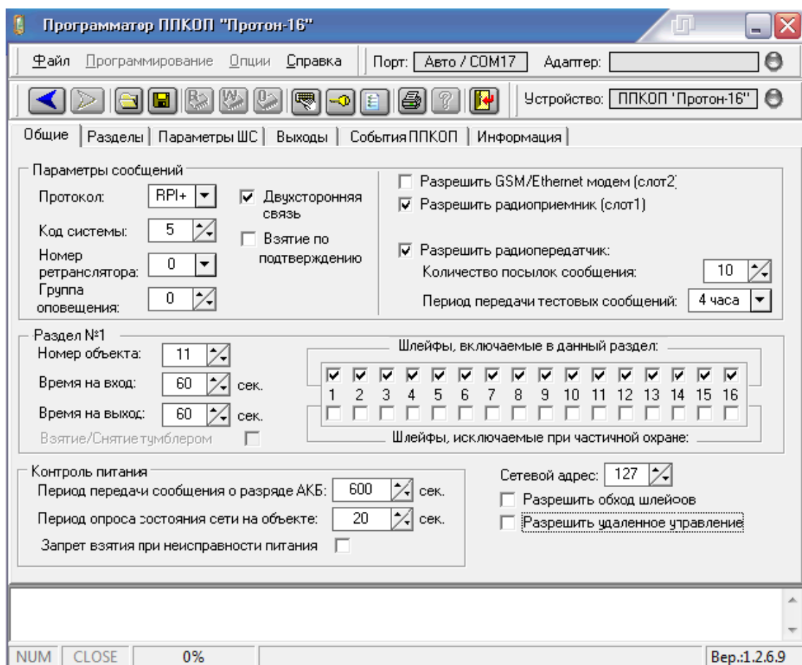
Рисунок 5 - Вкладка «Общие» программатора
