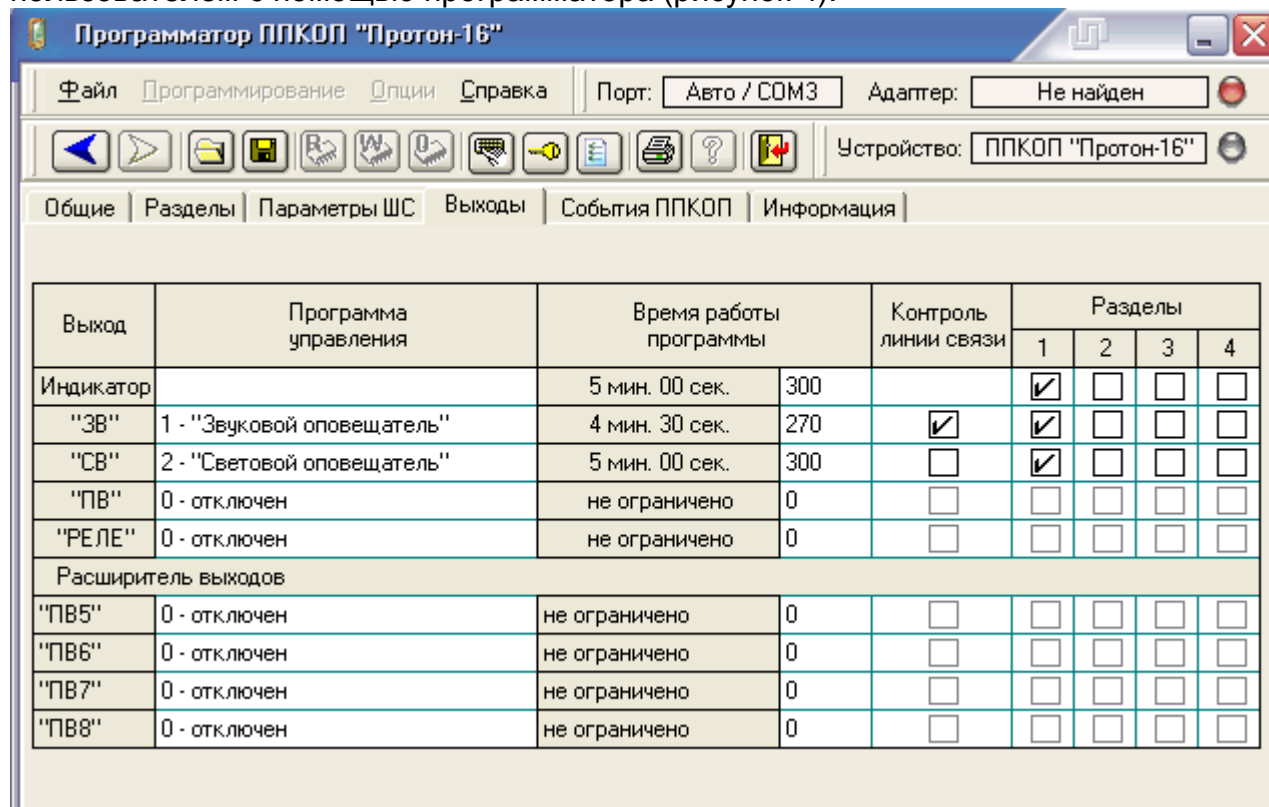
Рисунок 4 – Вкладка «Выходы» программатора
