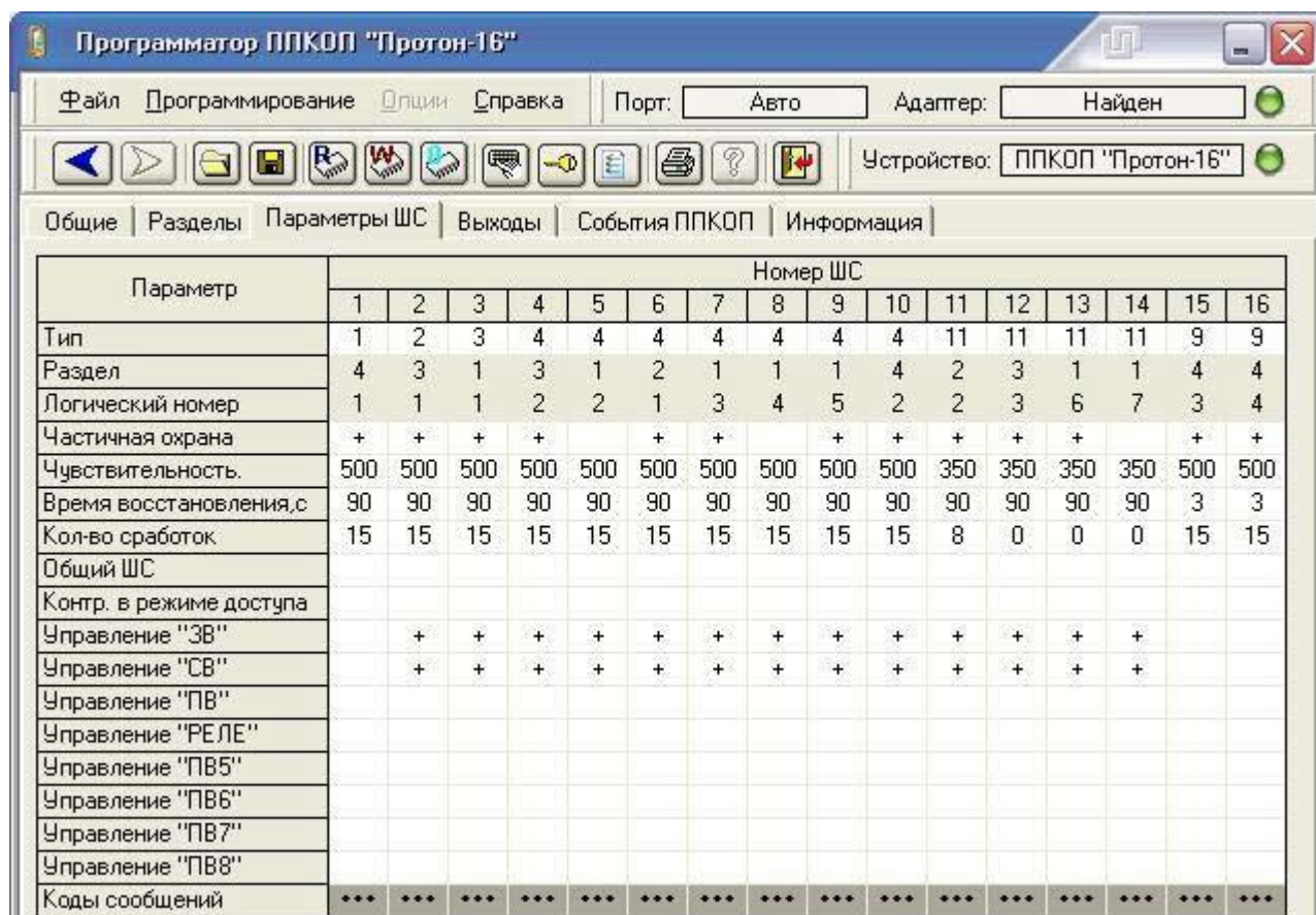
Рисунок 1 – вкладка «Параметры ШС» программатора
