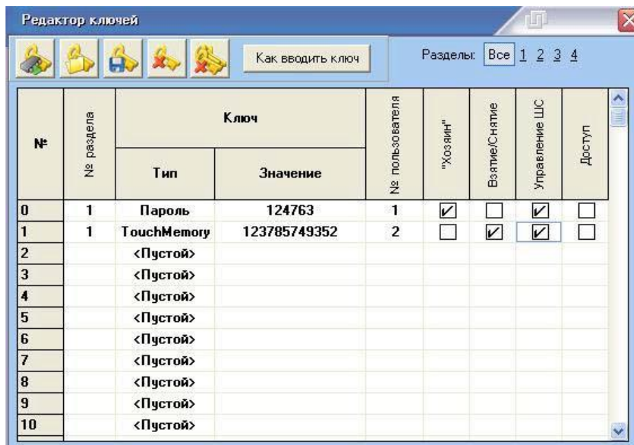
Рисунок 6 – Редактор ключей
