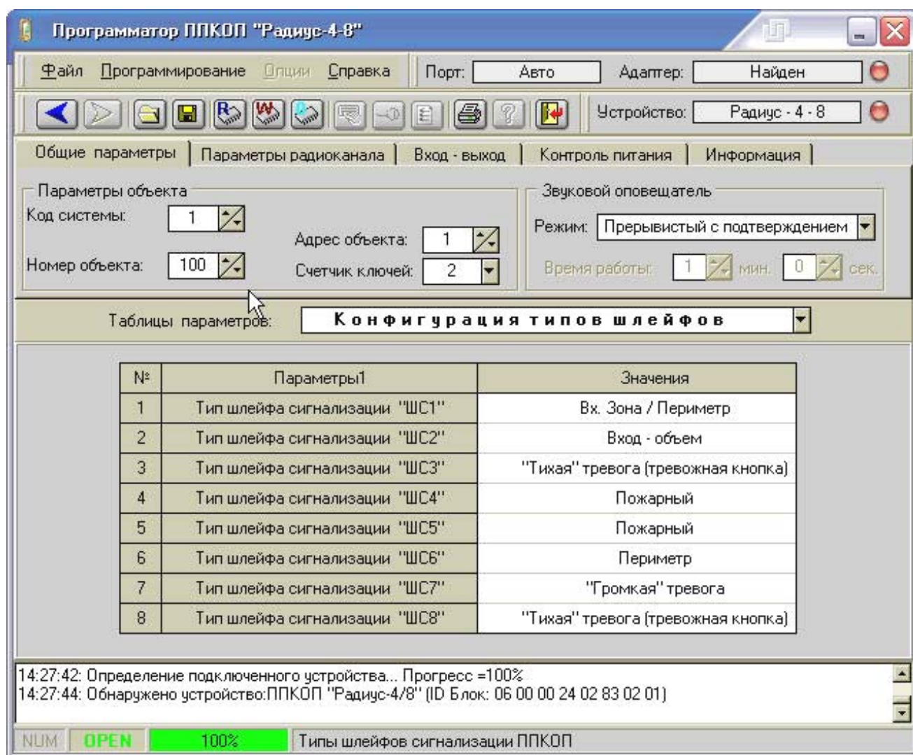
Рисунок 4 – Внешний вид оболочки программы
