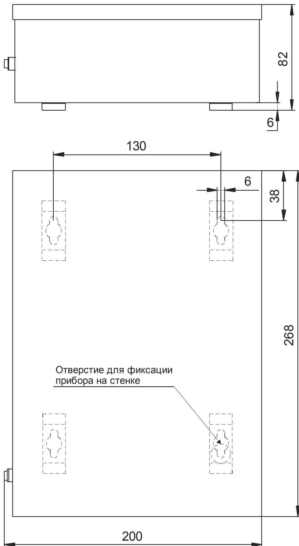
Рисунок А.1 - Габаритные и установочные размеры прибора «Радиус-4-И»
