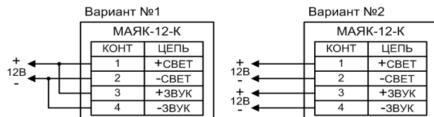
Рис.1 Схема подключения.
